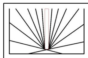
STAČIAKAMPIS
