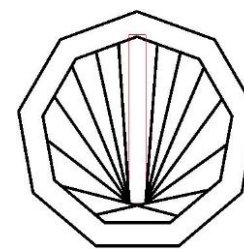
DEVYNKAMPIS
