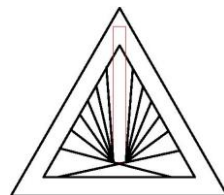
TRIKAMPIS
