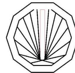
DEŠIMTKAMPIS
