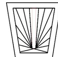
TRAPEZOIDAS
