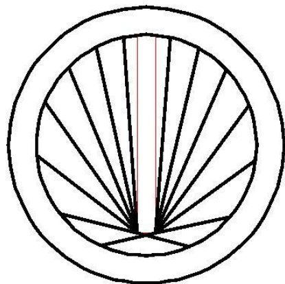
APSKRITIMAS
