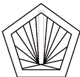
PENKIAKAMPIS
