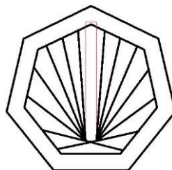
SEPTYNKAMPIS
