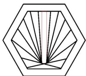
ŠEŠIAKAMPIS
