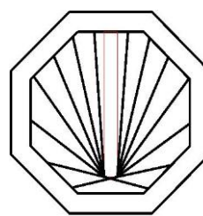
AŠTUONKAMPIS
