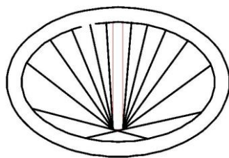
ELIPSĖ
