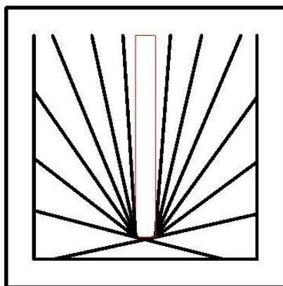
KVADRATAS
