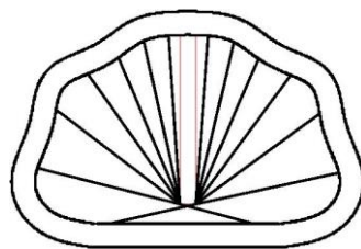
NETAISYKLINGA FORMA
